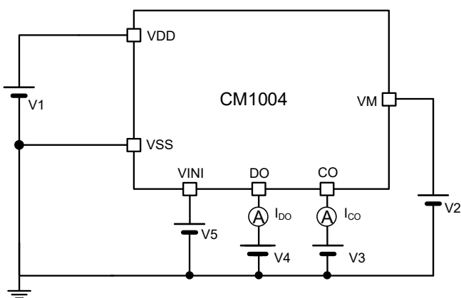
图 11 测试电路 4
