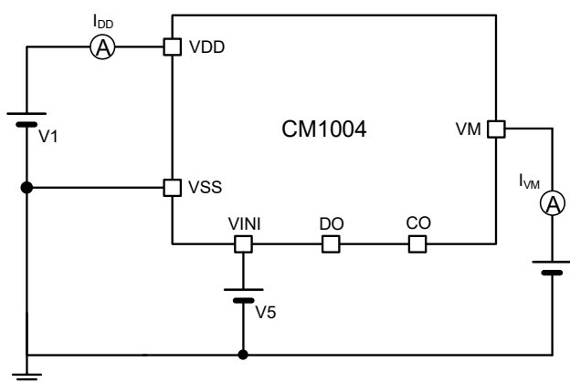
图 10 测试电路 3
