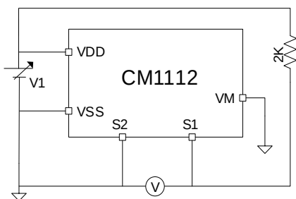
图 8 测试电路 1
