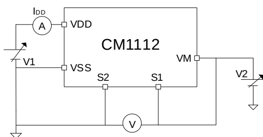
图 12 测试电路 5
