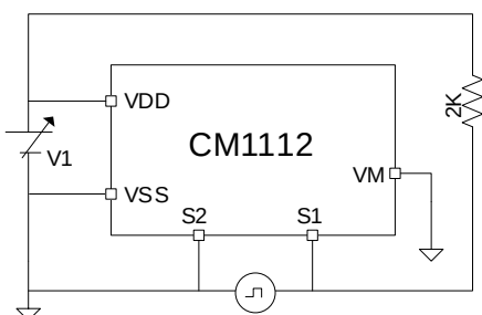
图 10 测试电路 3
